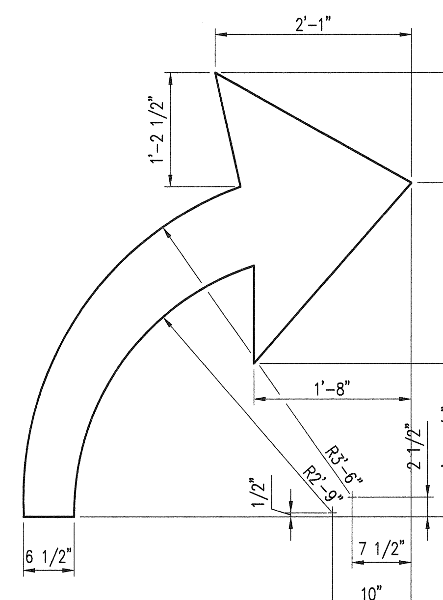
L-21 RIGHT ARROW NTS
