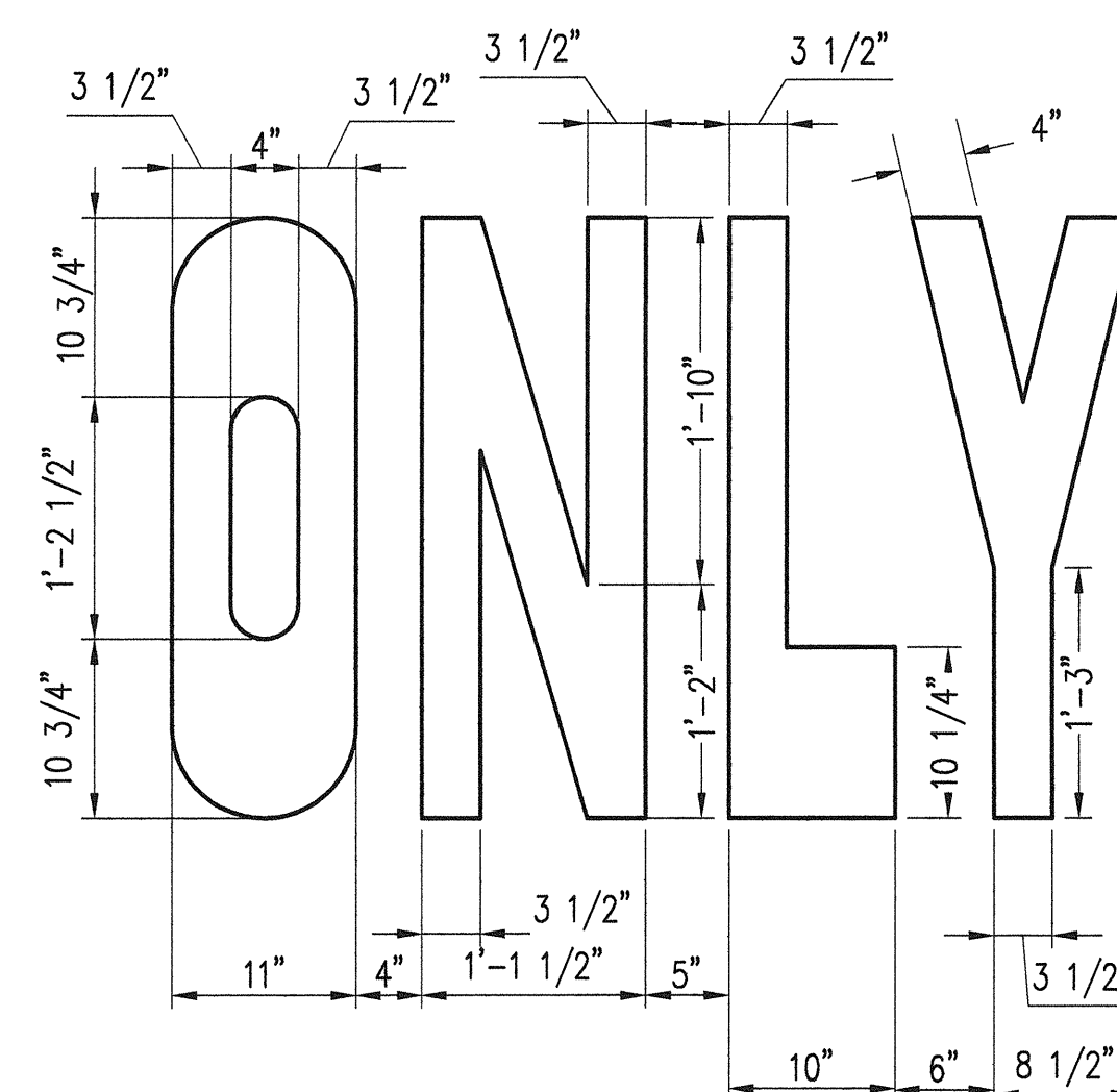
L-25 L-25T "ONLY" LEGEND NTS
