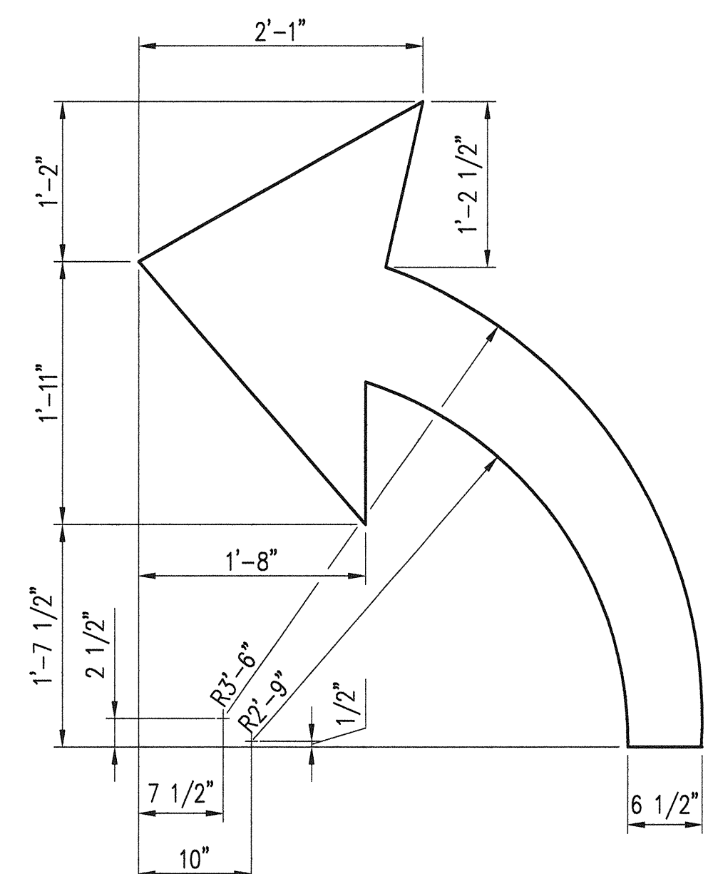
L-20 LEFT ARROW NTS
