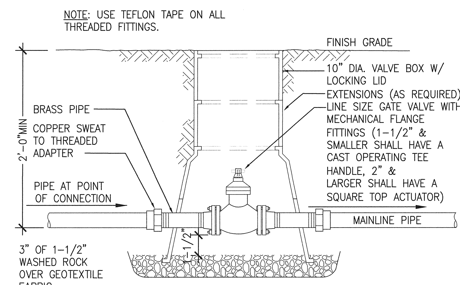
2 GATE VALVE SCALE: N.T.S. MC-GTVLV
