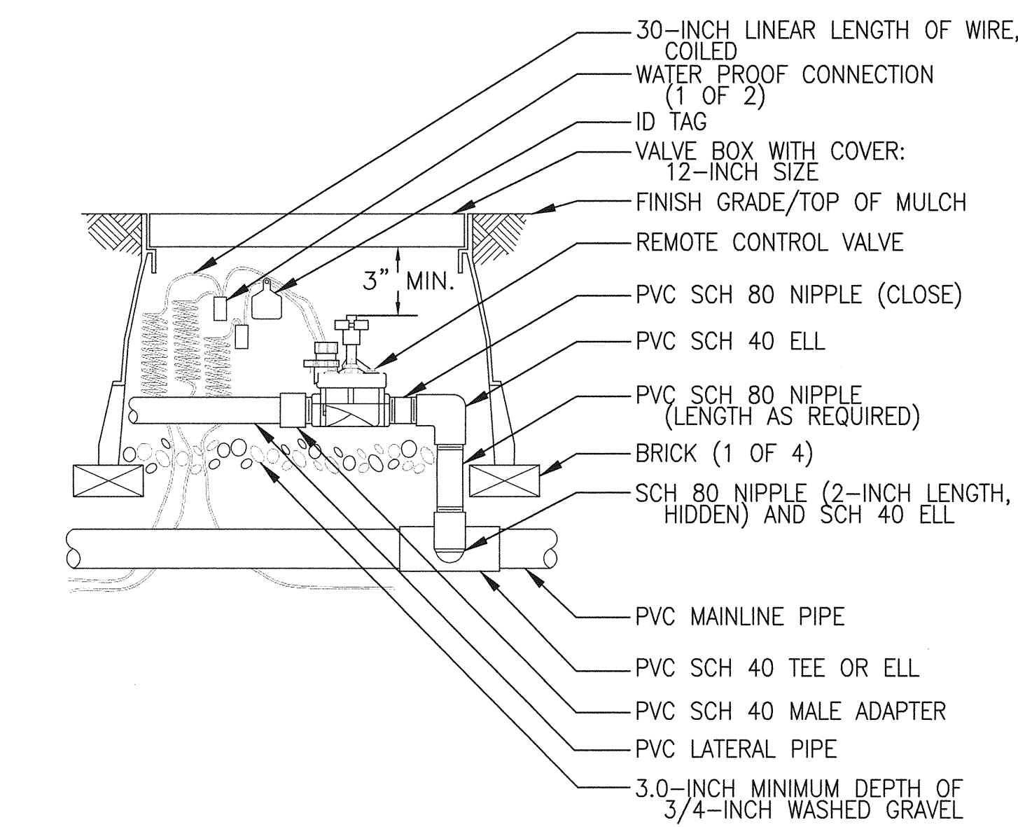
4 REMOTE CONTROL VALVE SCALE: N.T.S. MC-RC
