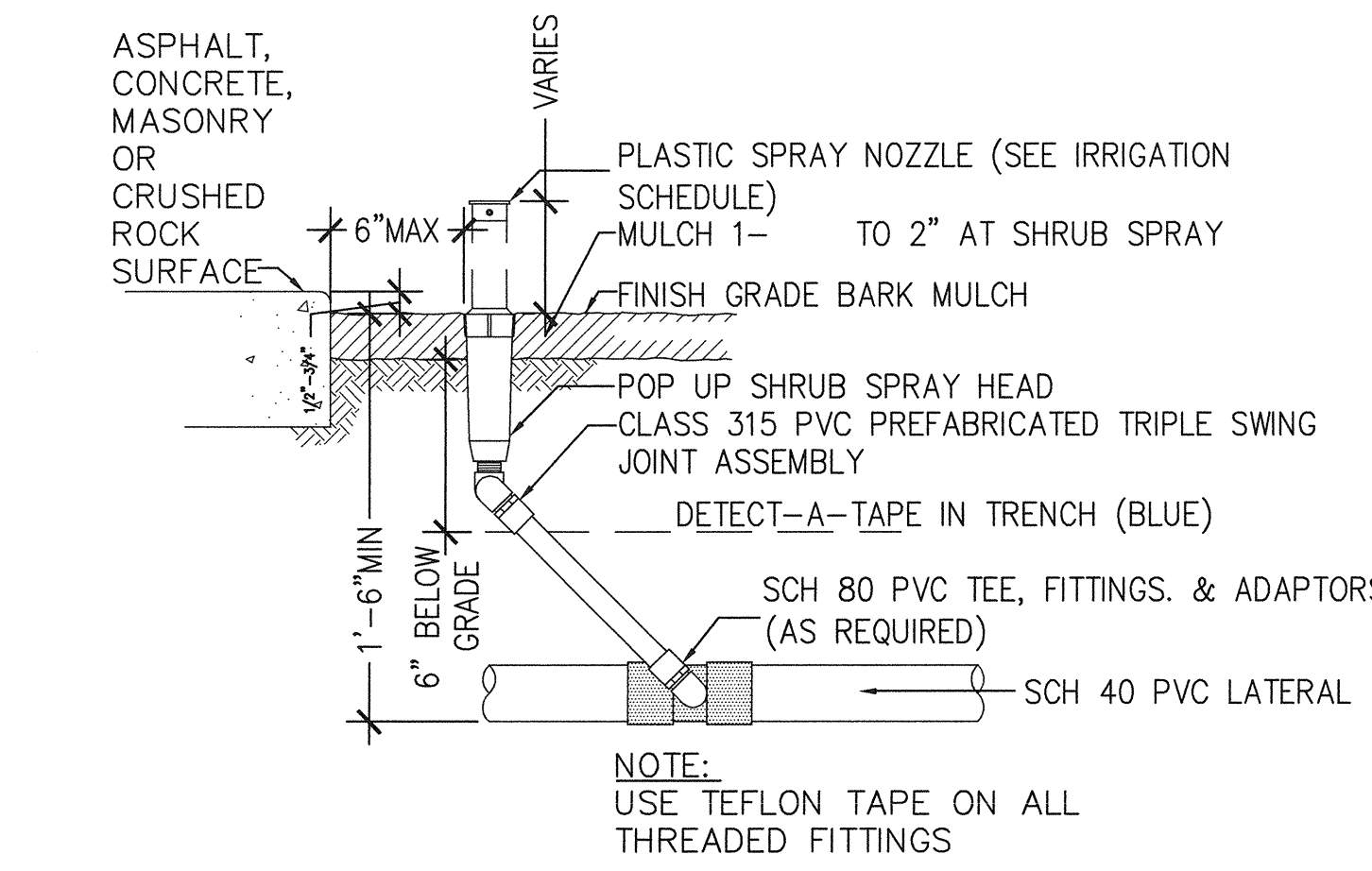
7 SPRAY HEAD SCALE: N.T.S. MC-SPR
