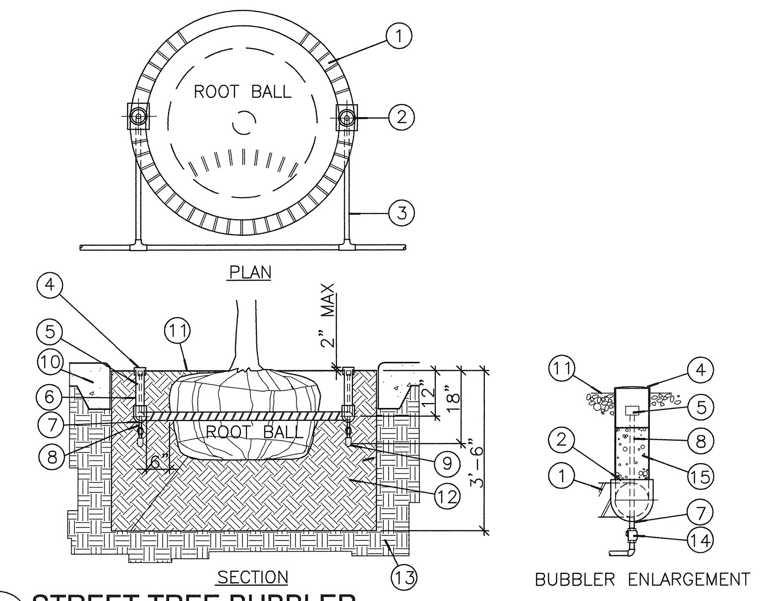
5 STREET TREE BUBBLER SCALE: N.T.S. MC-BUBBLER
