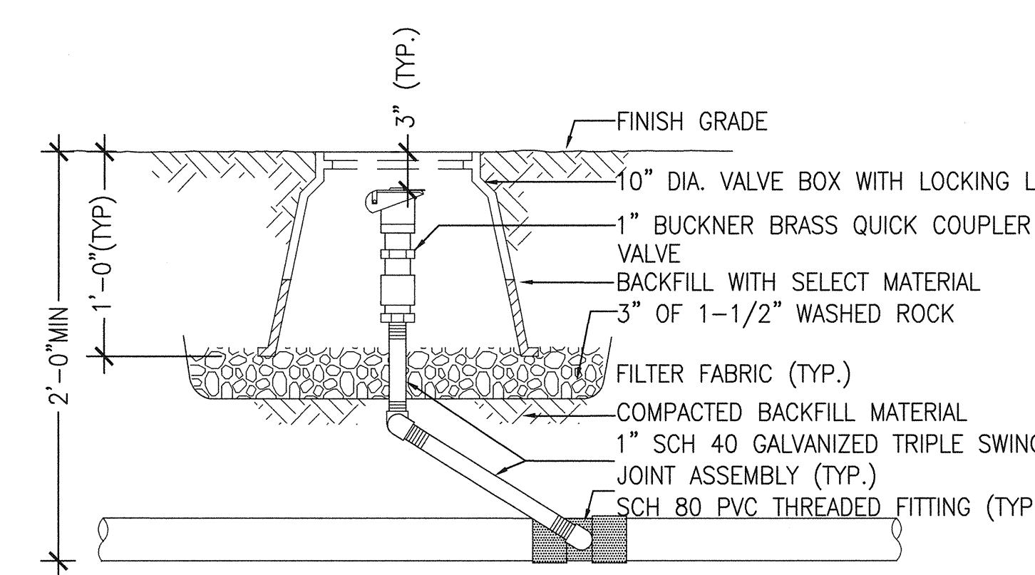
3 QUICK COUPLER VALVE SCALE: N.T.S. MC-QCV
