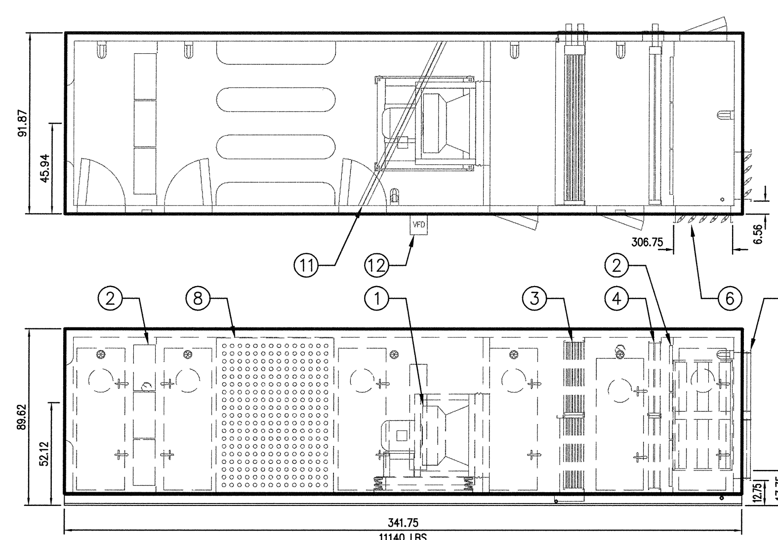
AHU-1 SCALE: 1/4"=1'-0"
