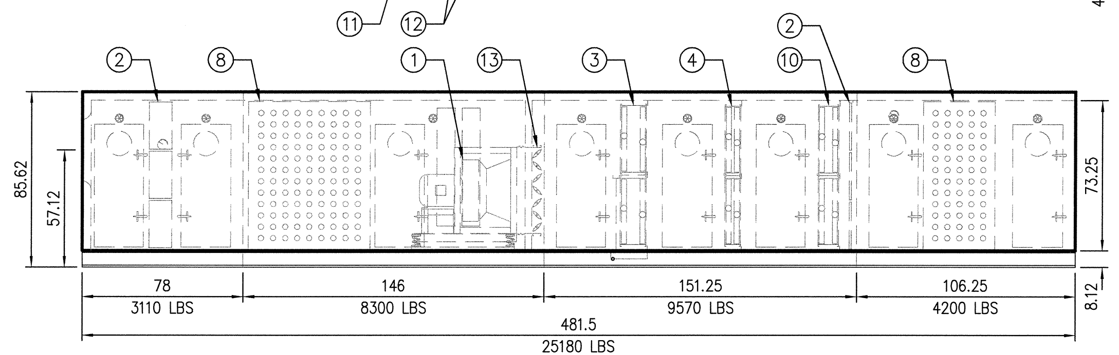
AHU-2 SCALE: 1/4"=1'-0"
