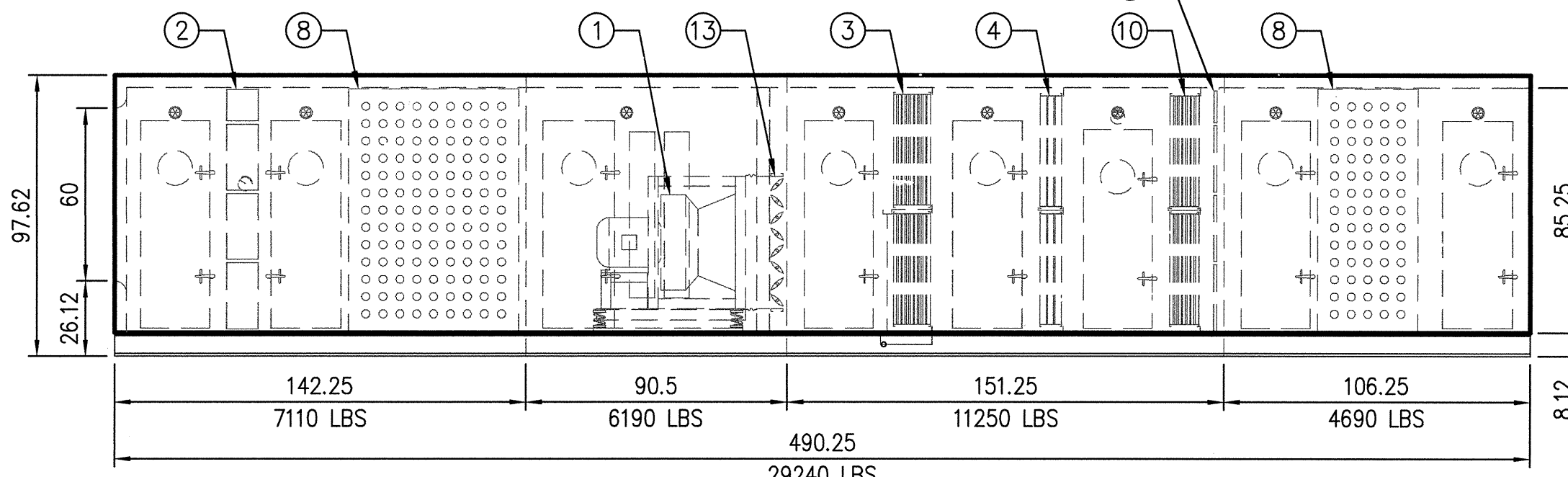
AHU-3 SCALE: 1/4"=1'-0"
