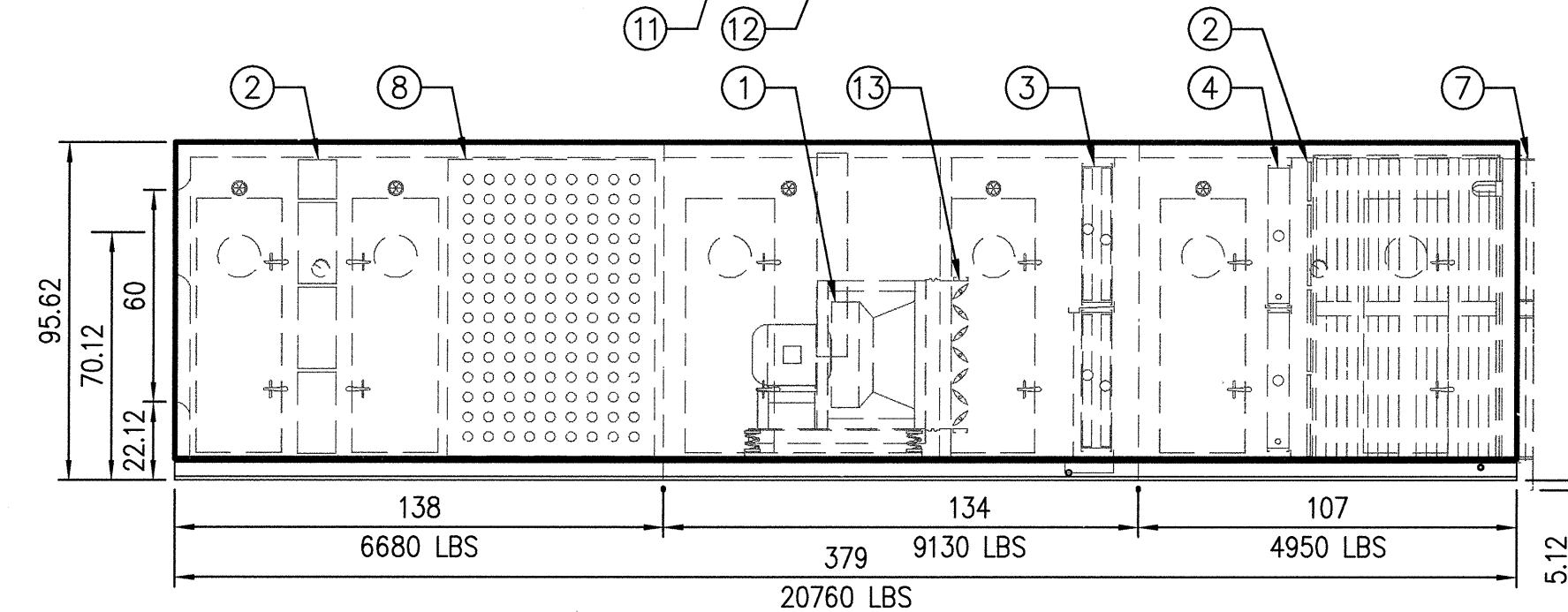
AHU-4 SCALE: 1/4"=1'-0"
