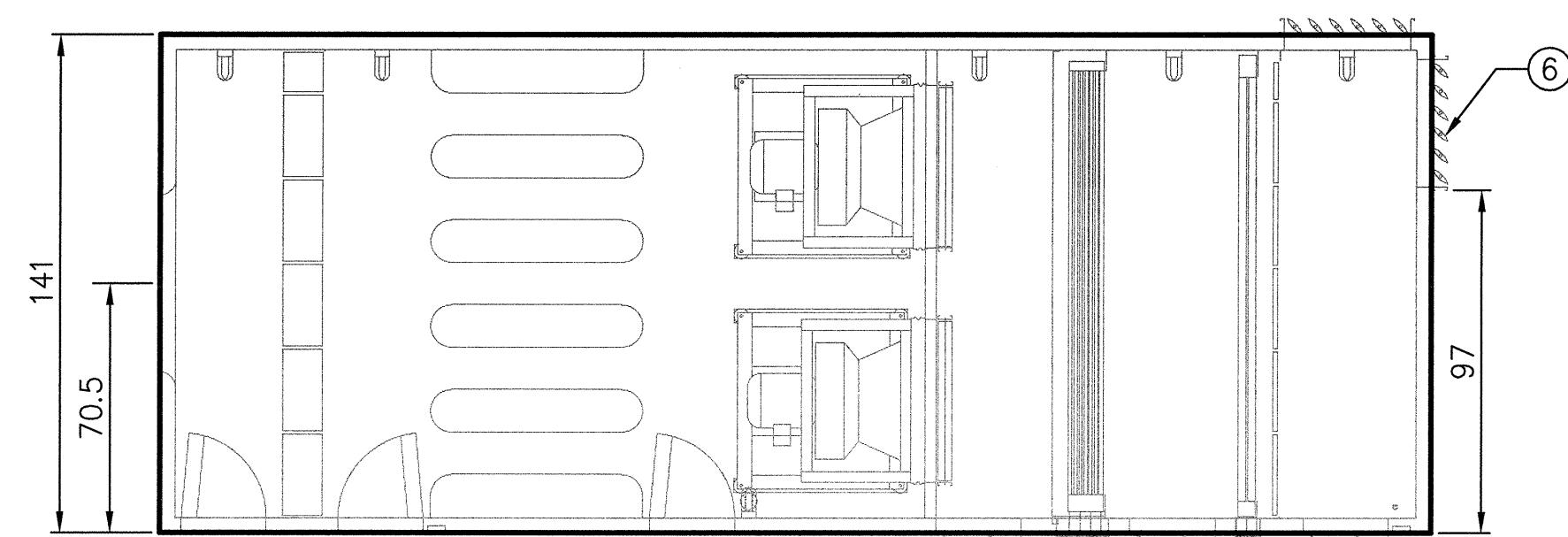
AHU-4 SCALE: 1/4"=1'-0"
