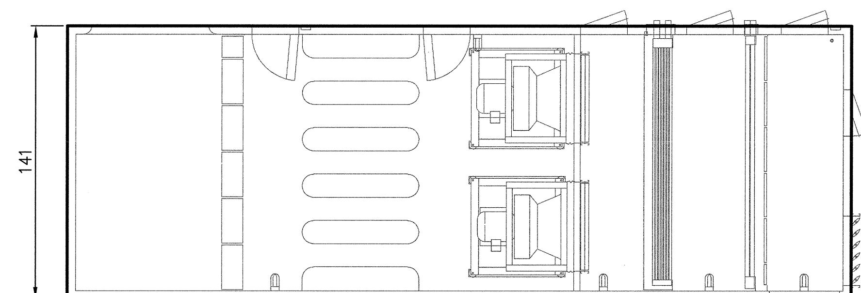
FUTURE AHU-6 SCALE: 1/4"=1'-0"
