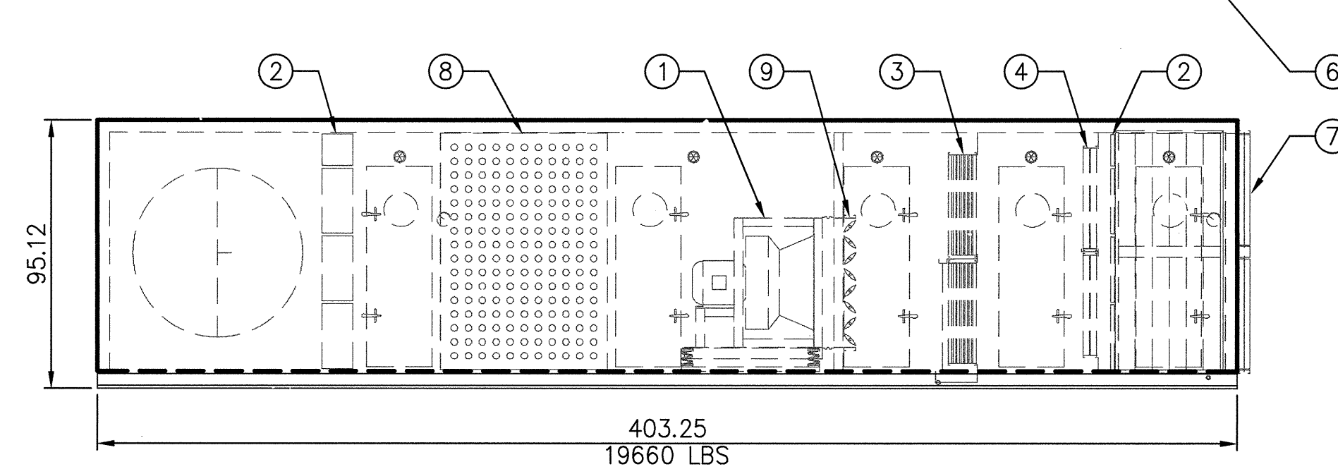
FUTURE AHU-7 SCALE: 1/4"=1'-0"
