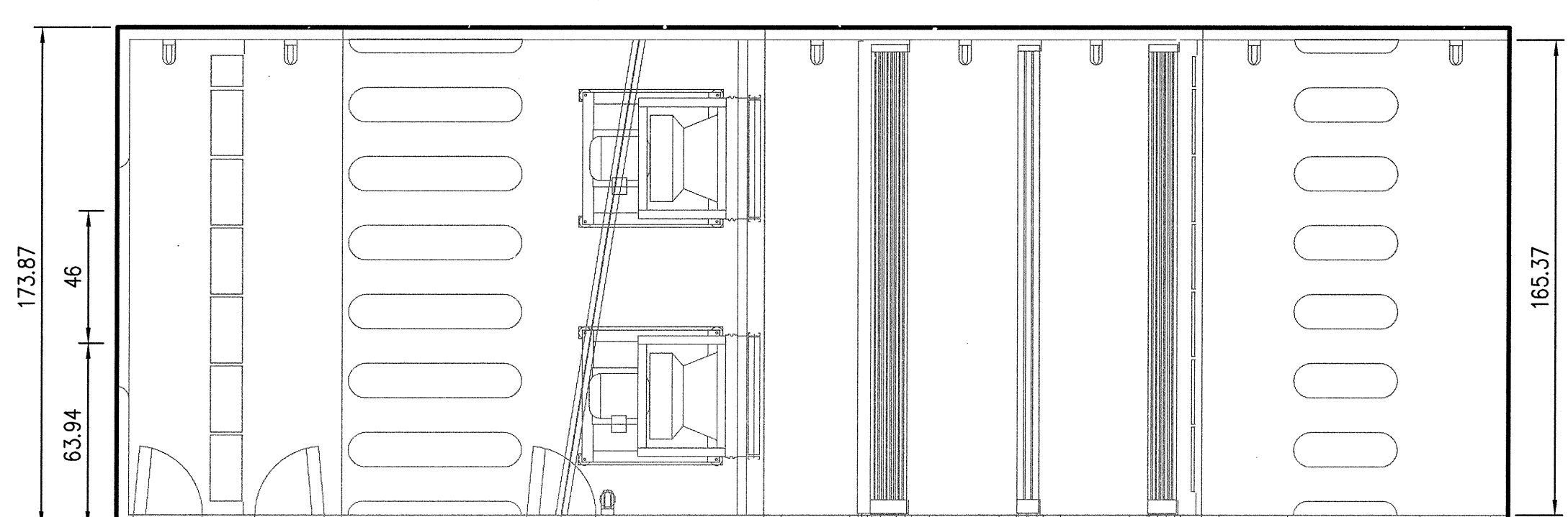
AHU-1 SCALE: 1/4"=1'-0"
