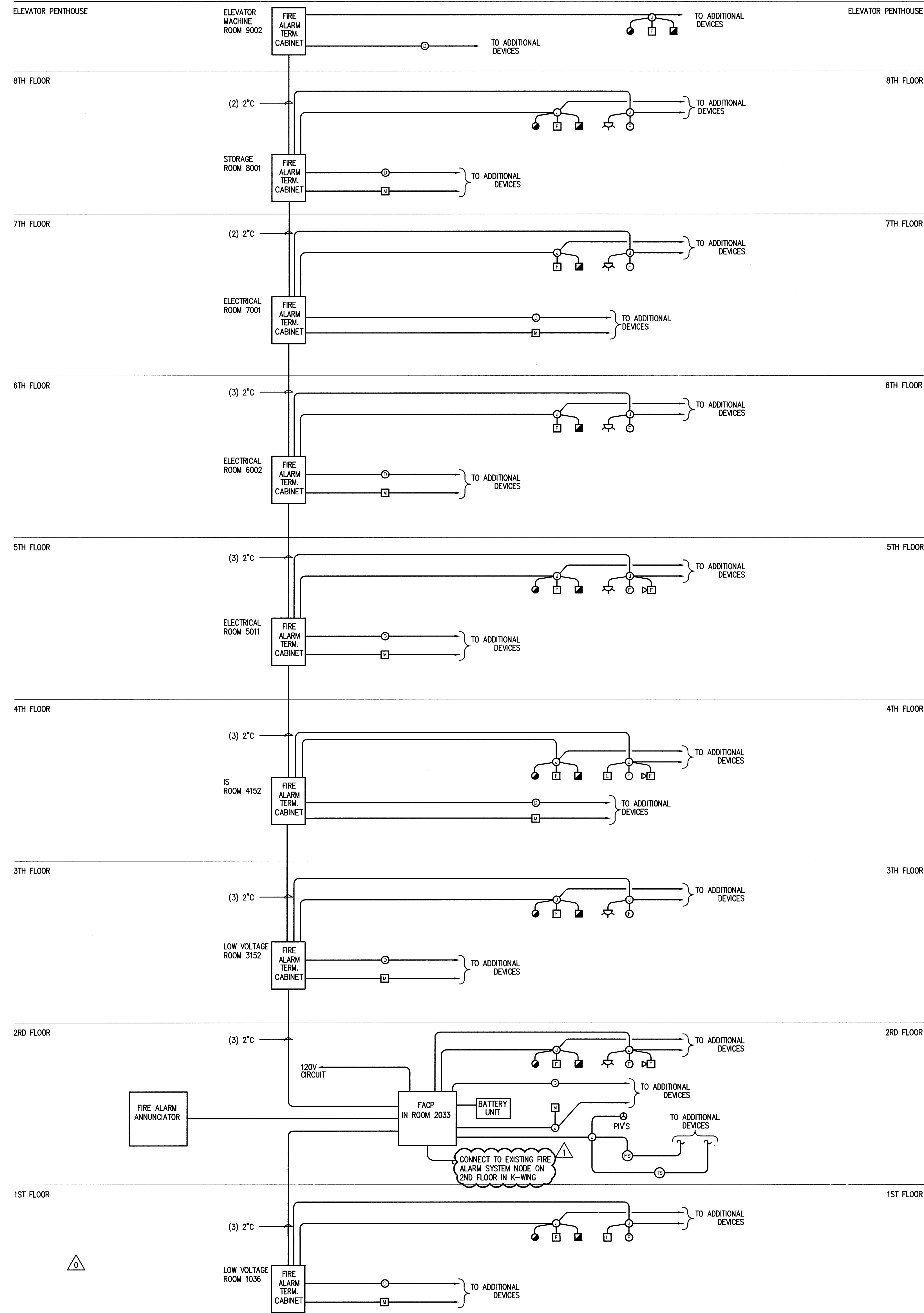
1 ONE-LINE / RISER DIAGRAM - FA RISER E6.05 SCALE: NONE
