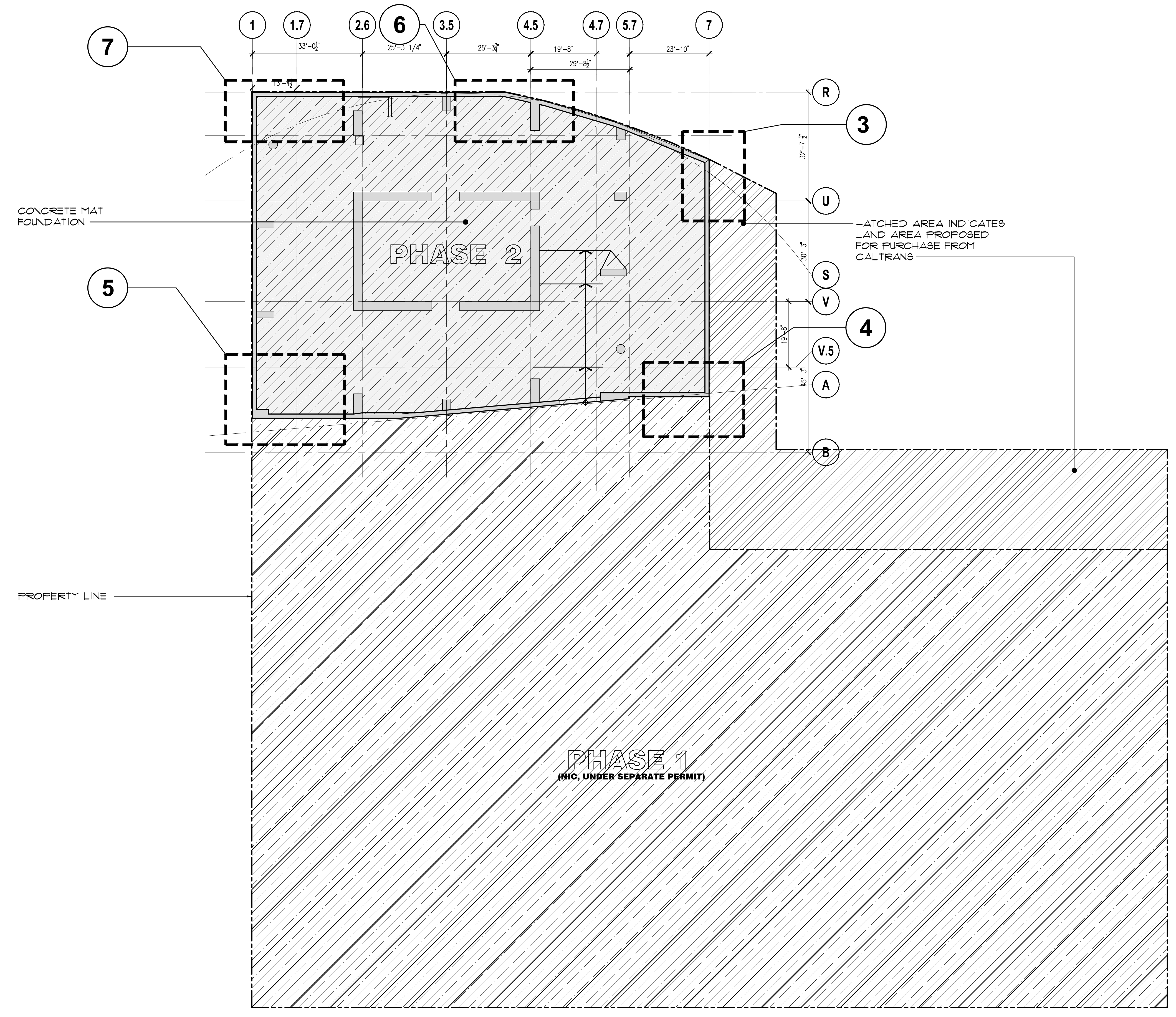
2 SCALE: 1/16" = 1'-0"
