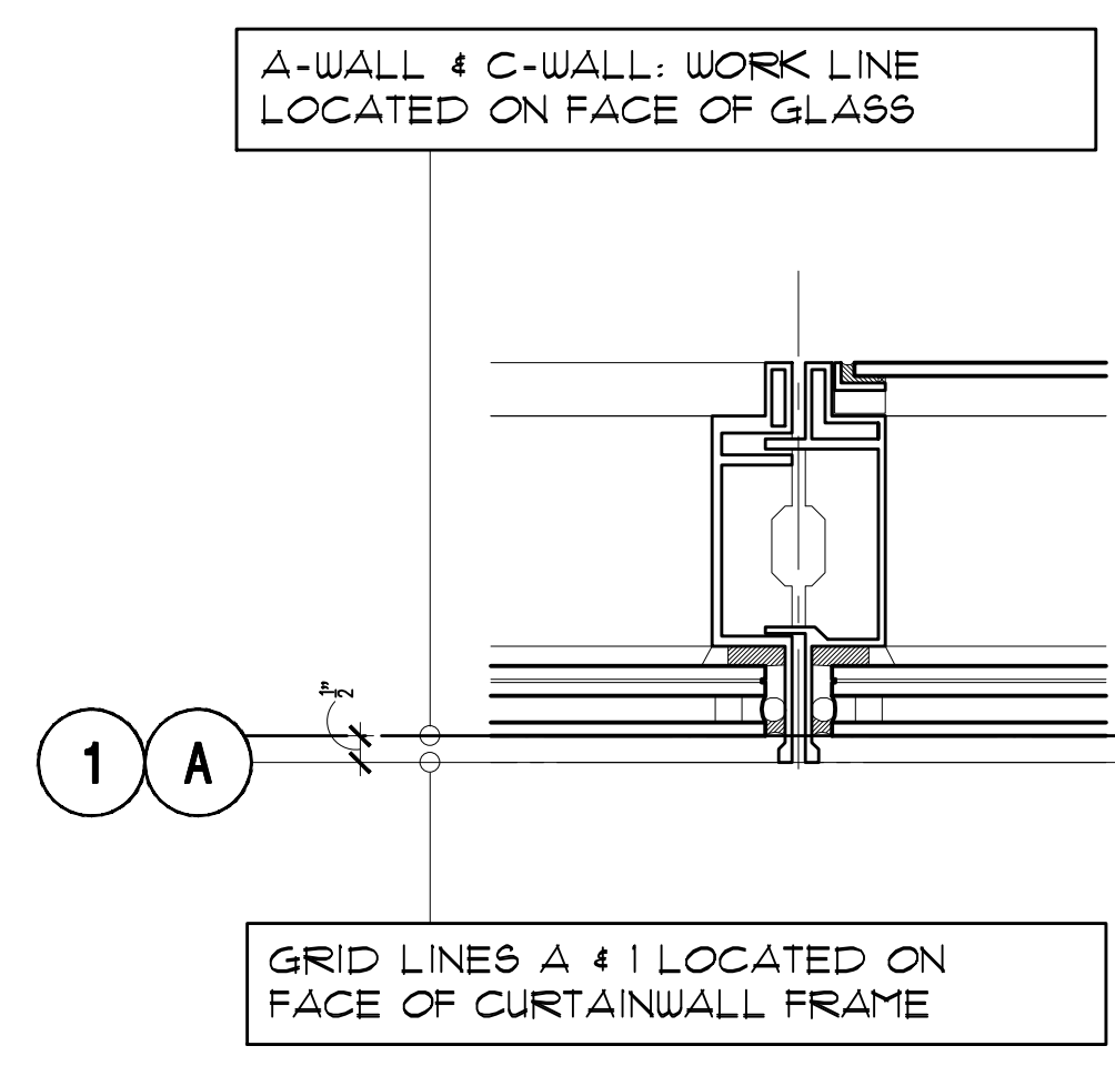
3 A-WALL C-WALL DETAIL SCALE: 3" = 1'-0"
