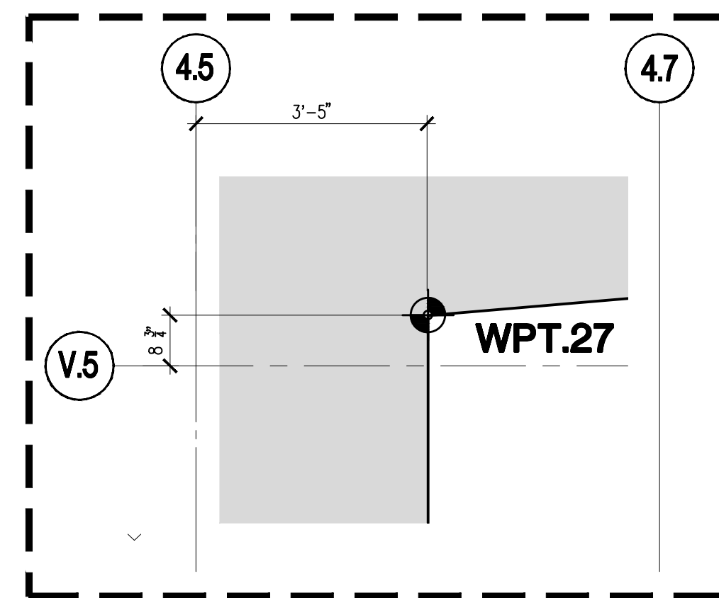
9 SCALE: 1/2" = 1'-0"
