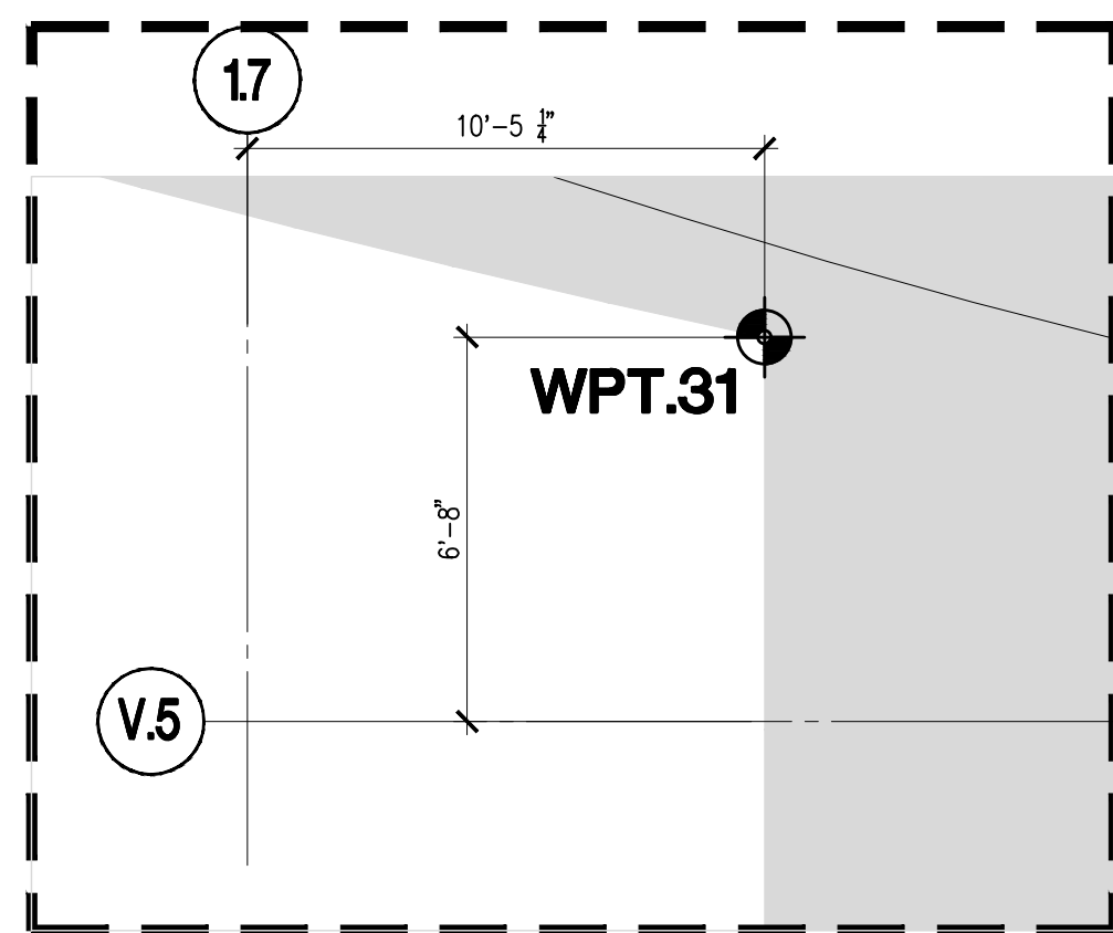
13 SCALE: 1/2" = 1'-0"
