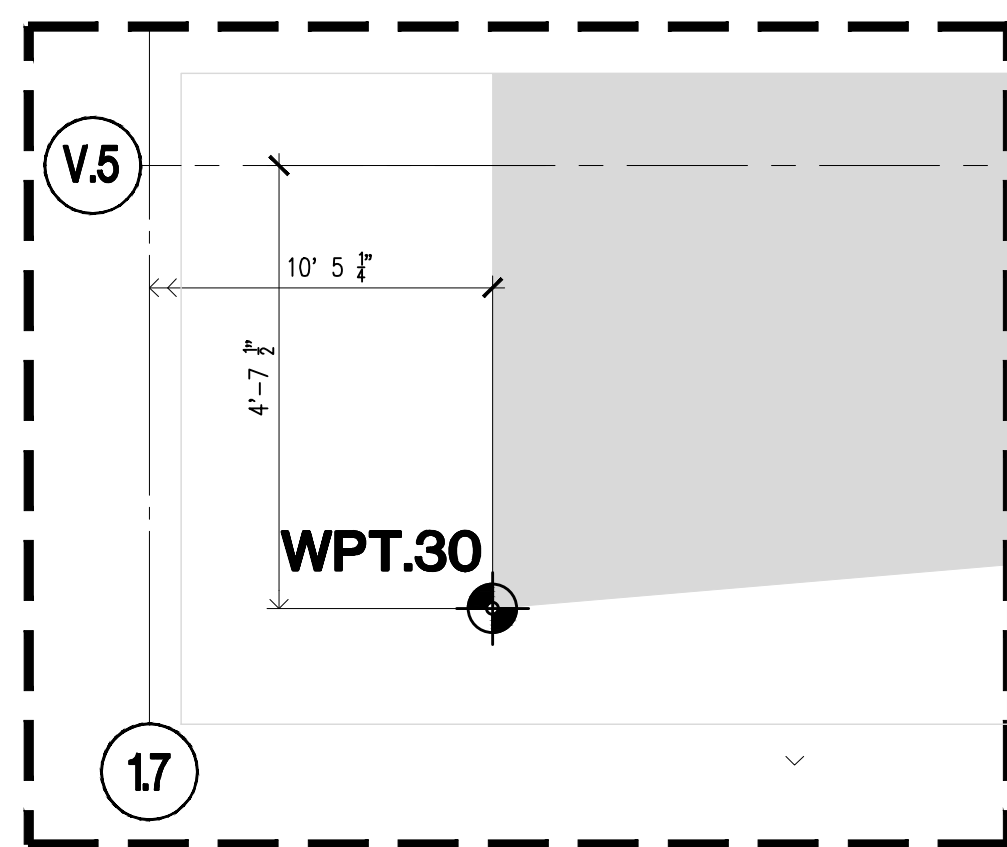
14 SCALE: 1/2" = 1'-0"
