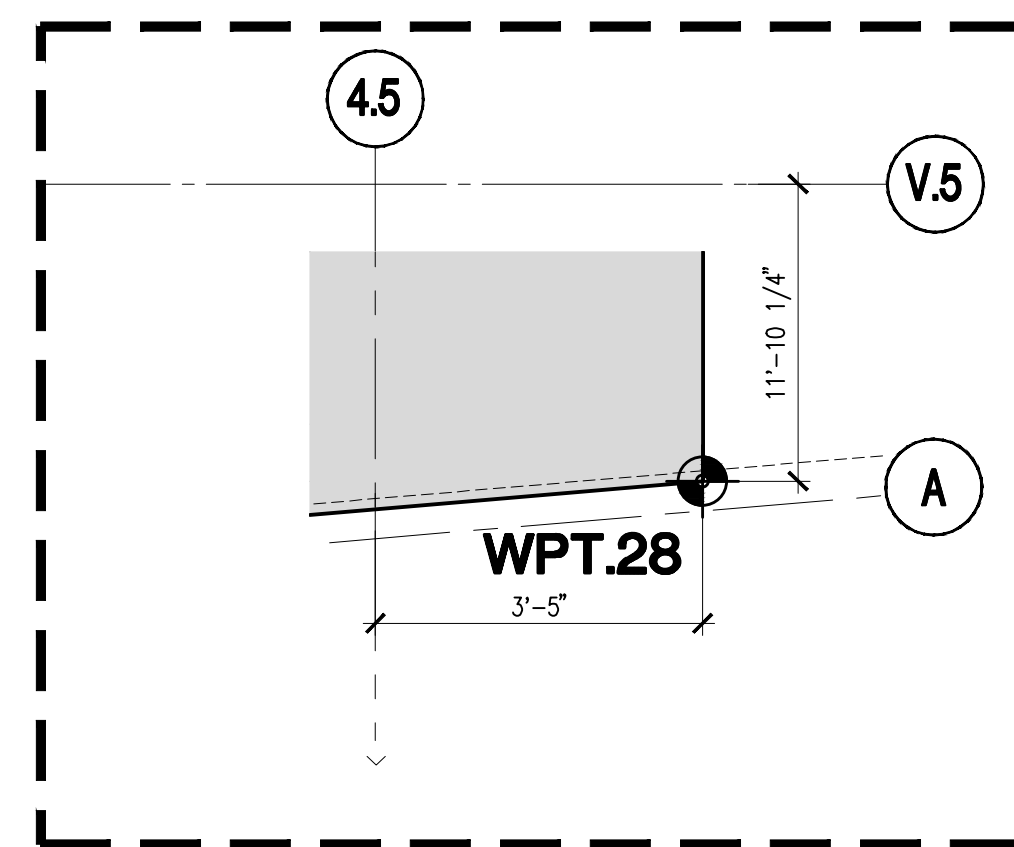
10 SCALE: 1/2" = 1'-0"
