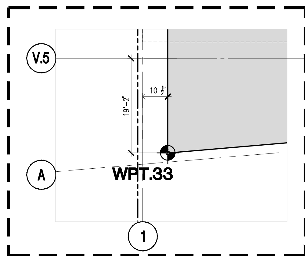
11 SCALE: 1/2" = 1'-0"
