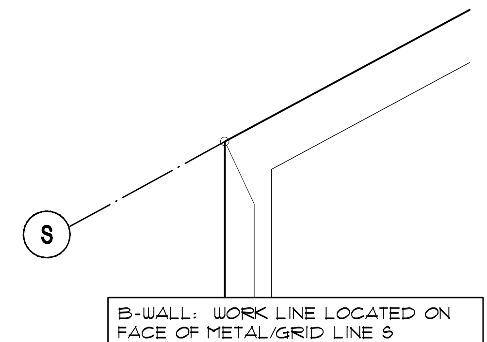
4 B-WALL DETAIL SCALE: 3" = 1'-0"
