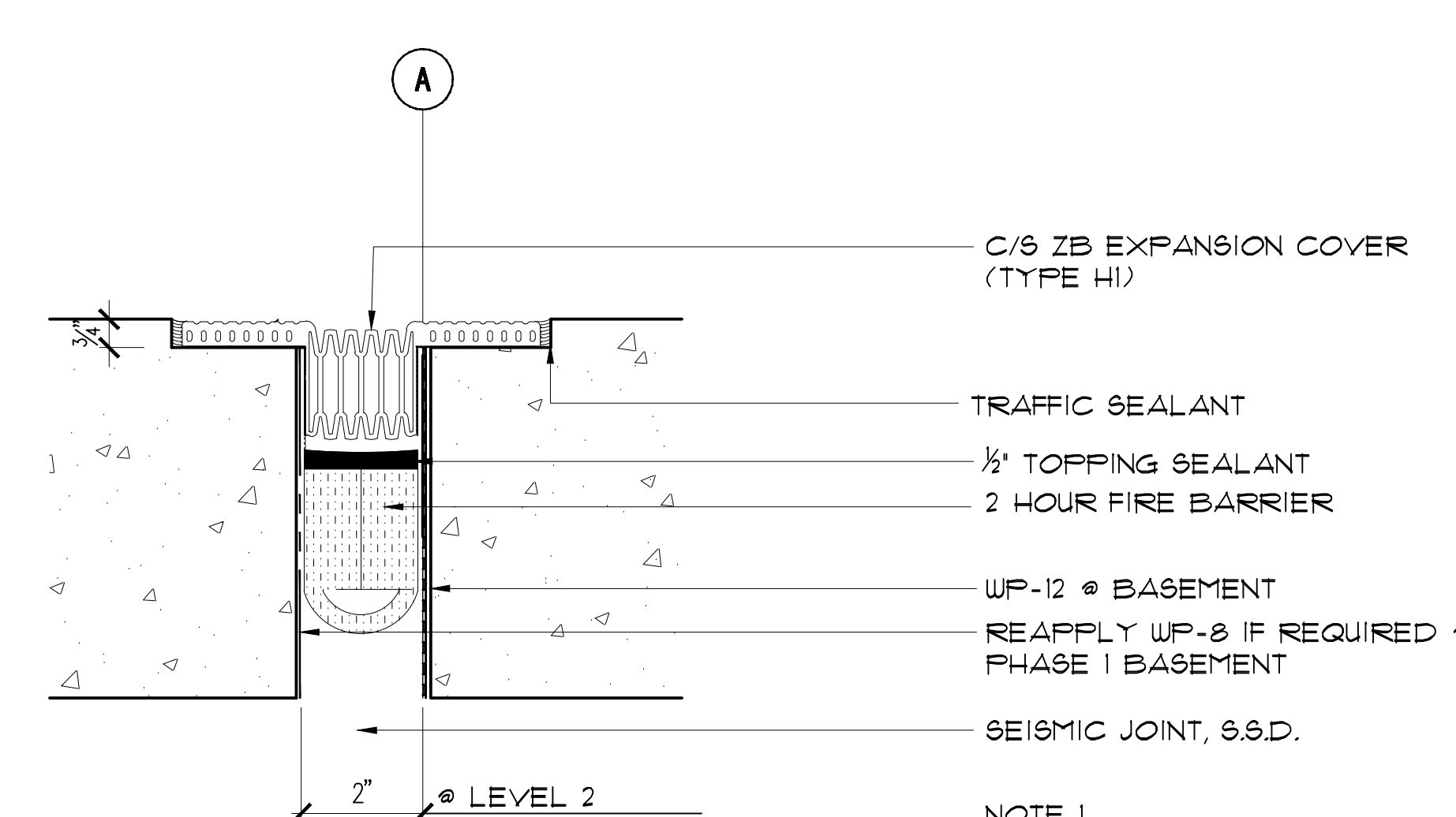
1 E.J. COVER (TYPE H1) SCALE: 3" = 1'-0"
