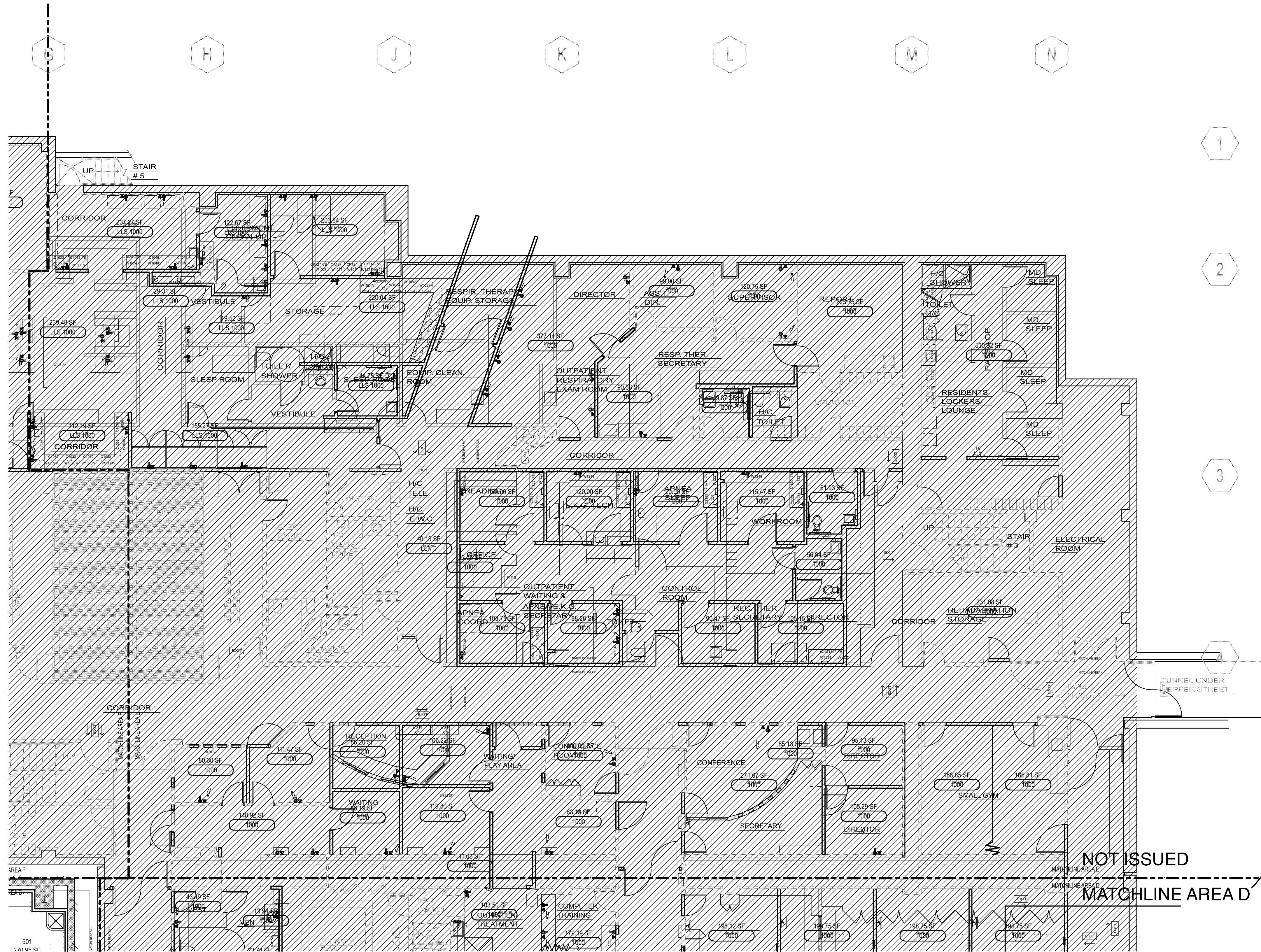
B6 FINISH PLAN SCALE: 1/8" = 1'-0"
