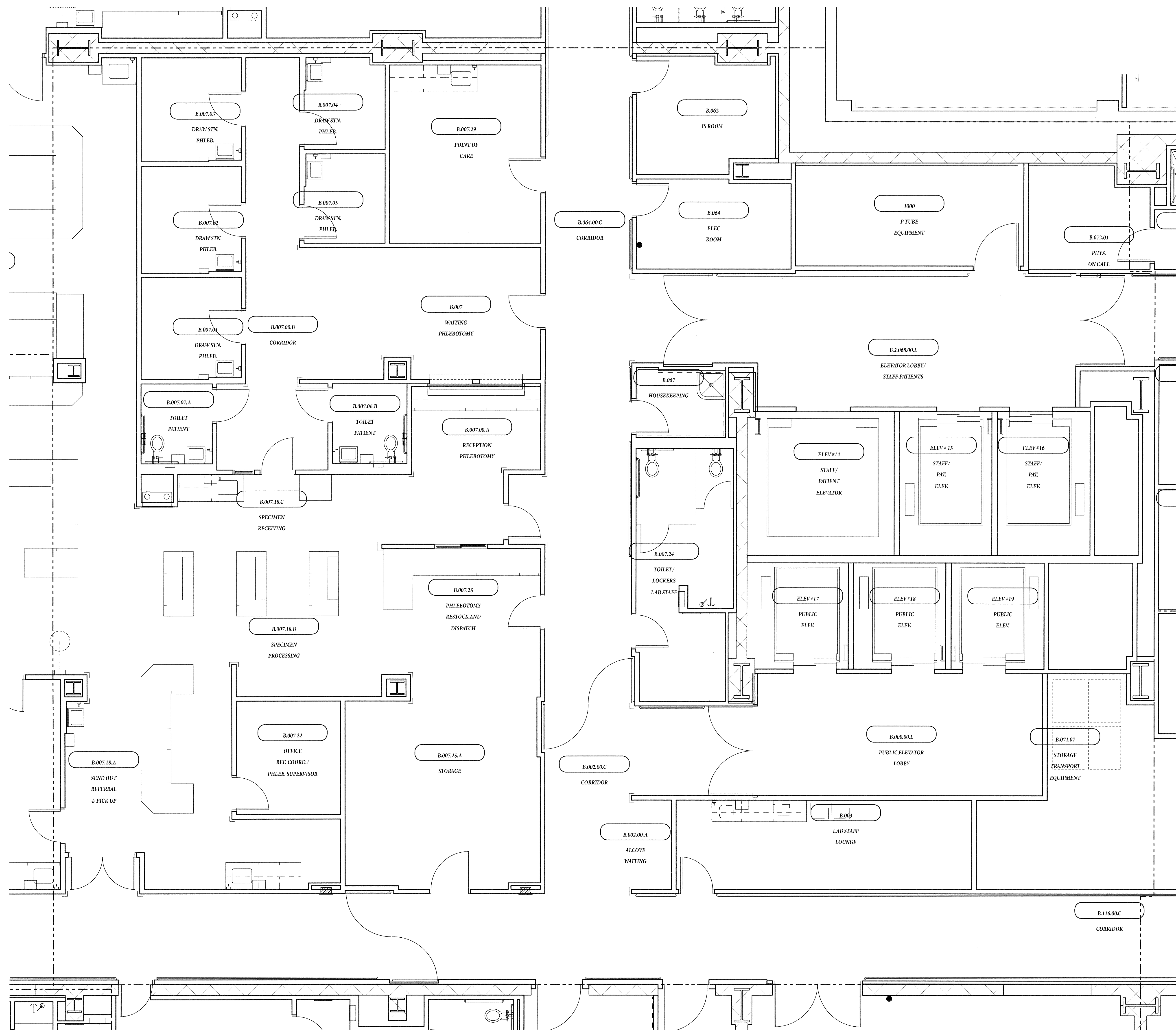
A6 Furniture Plan SCALE: 1/8" = 1'-0"
