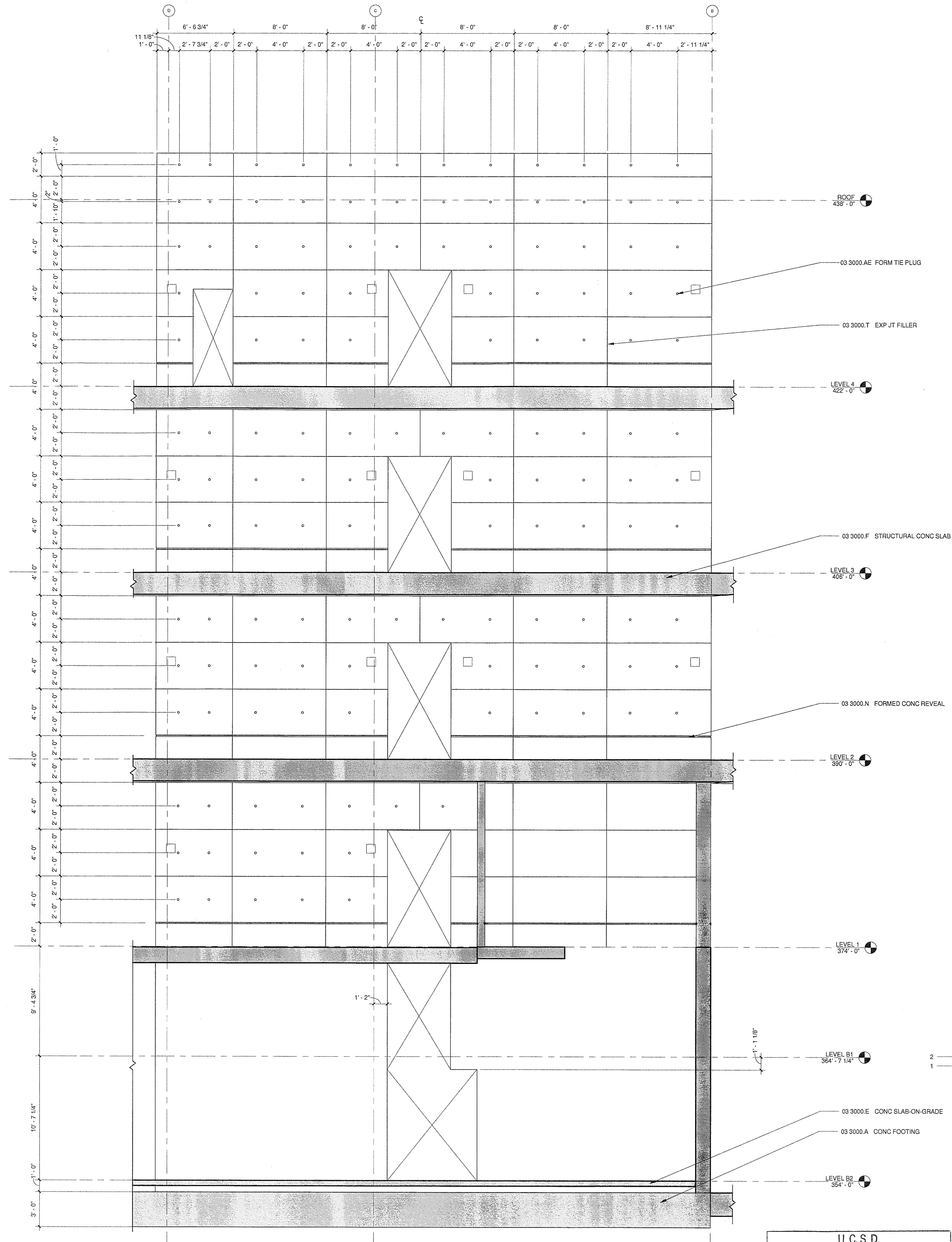
1 EXTERIOR CONC. WALL ELEV. A2511/A5306 1/4" = 1'-0"
