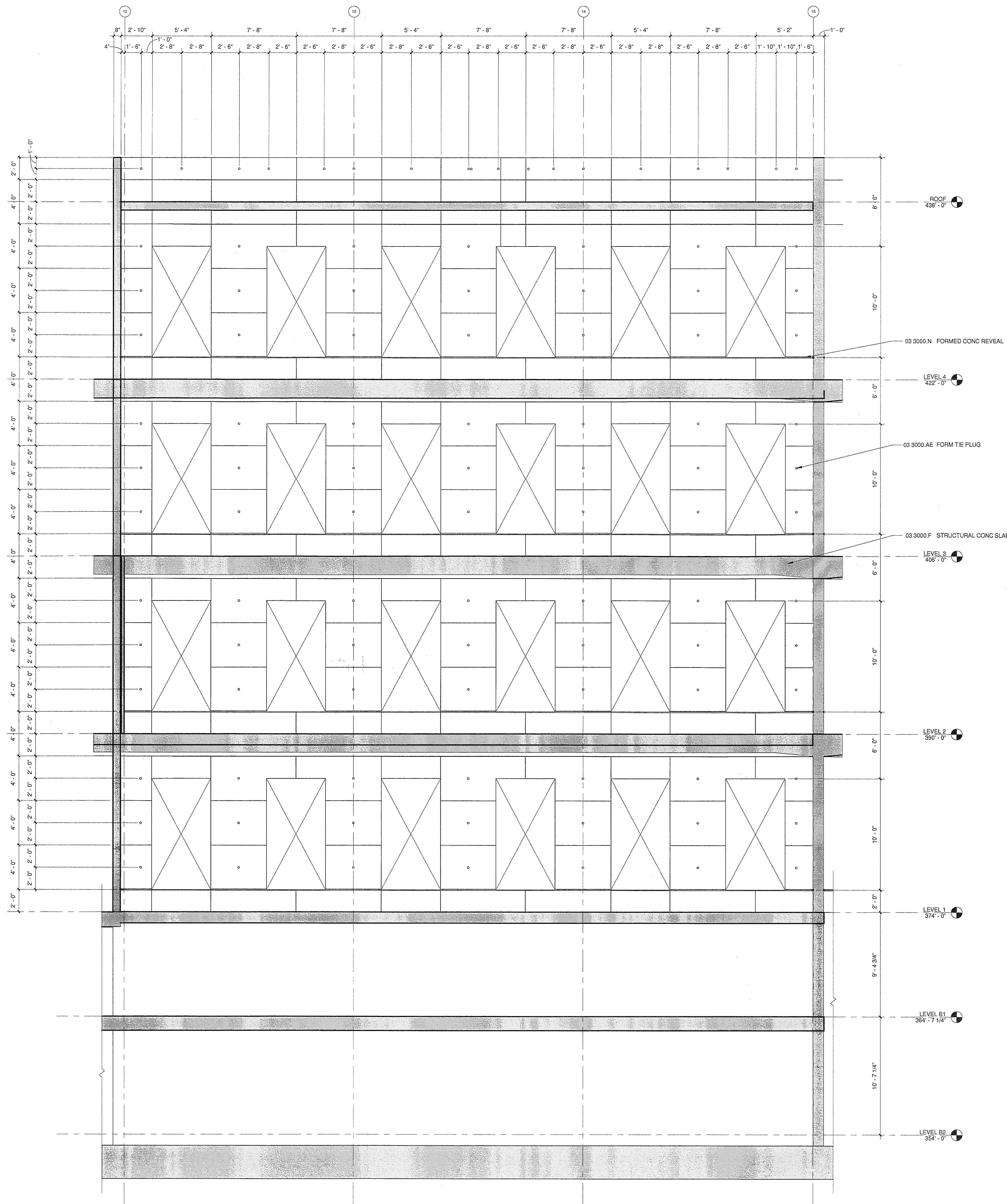
2 INTERIOR CONC. WALL ELEV. A5311 A5313 1/4" = 1'-0"
