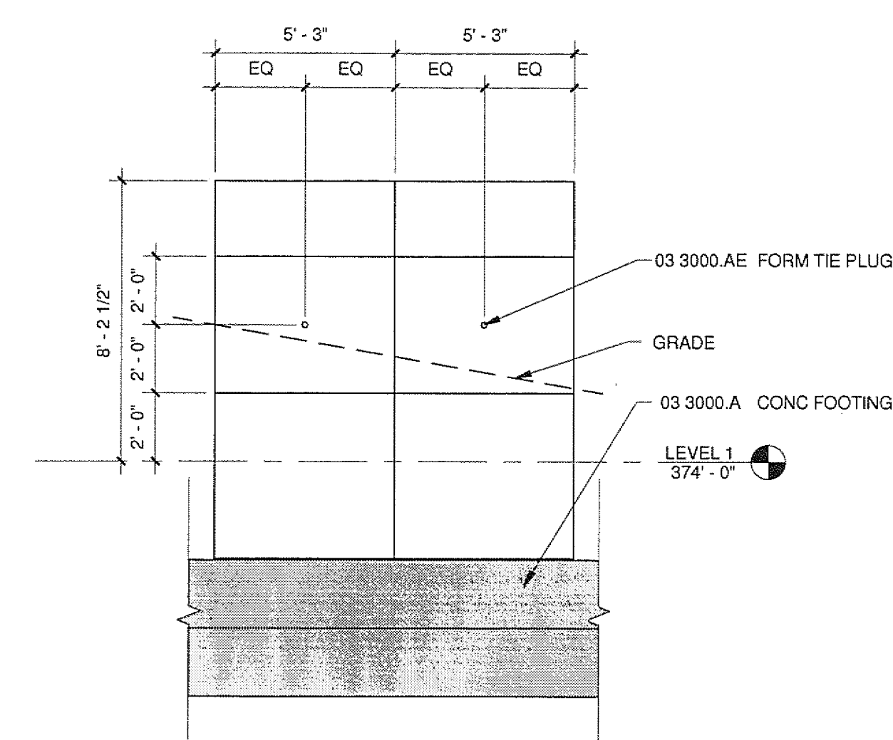
24 EXTERIOR CONC. WALL ELEV. A2515 | A5320 1/4" = 1'-0"
