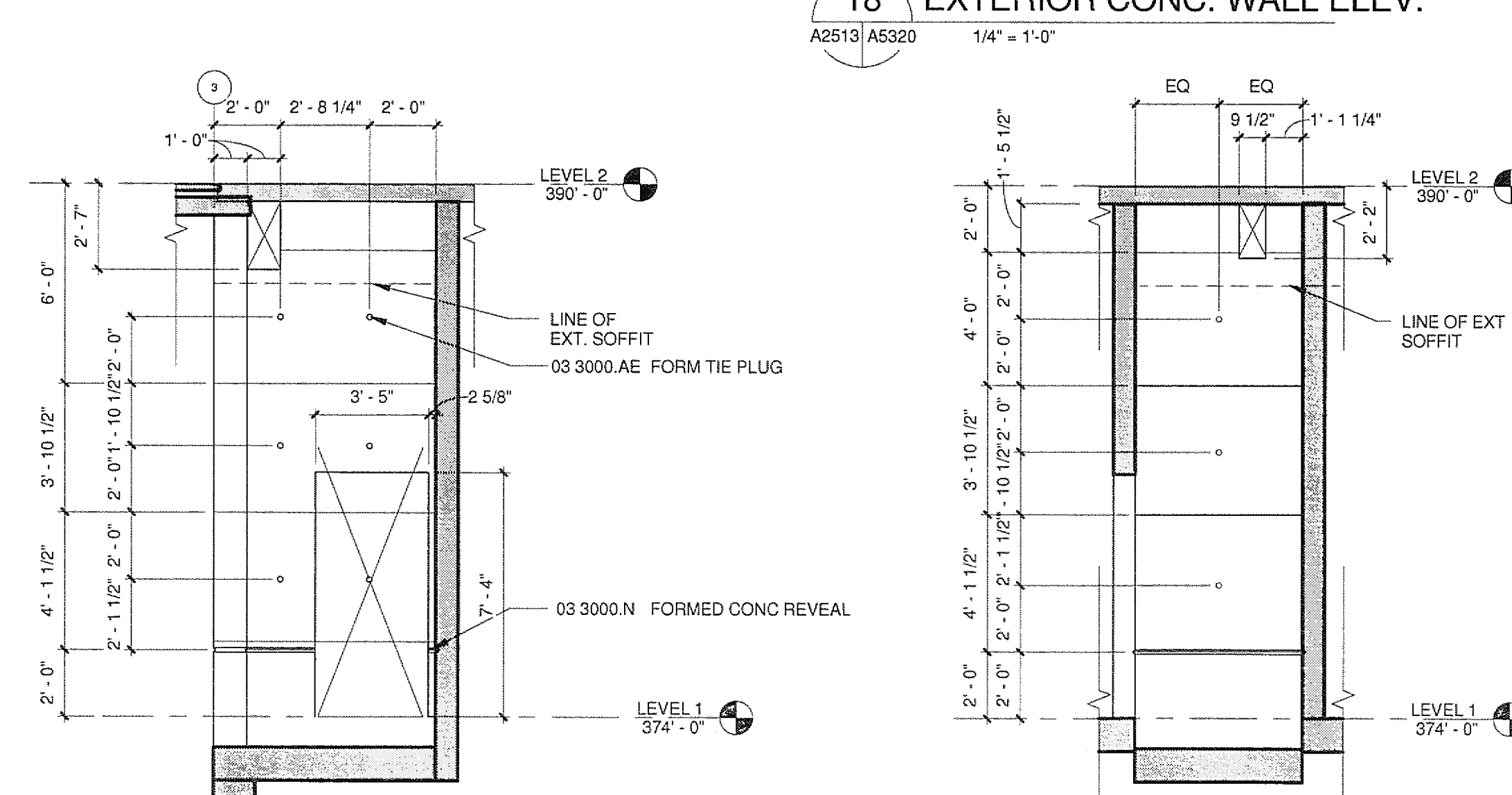
21 EXTERIOR CONC. WALL ELEV. A2513 A5320 1/4" = 1'-0"
