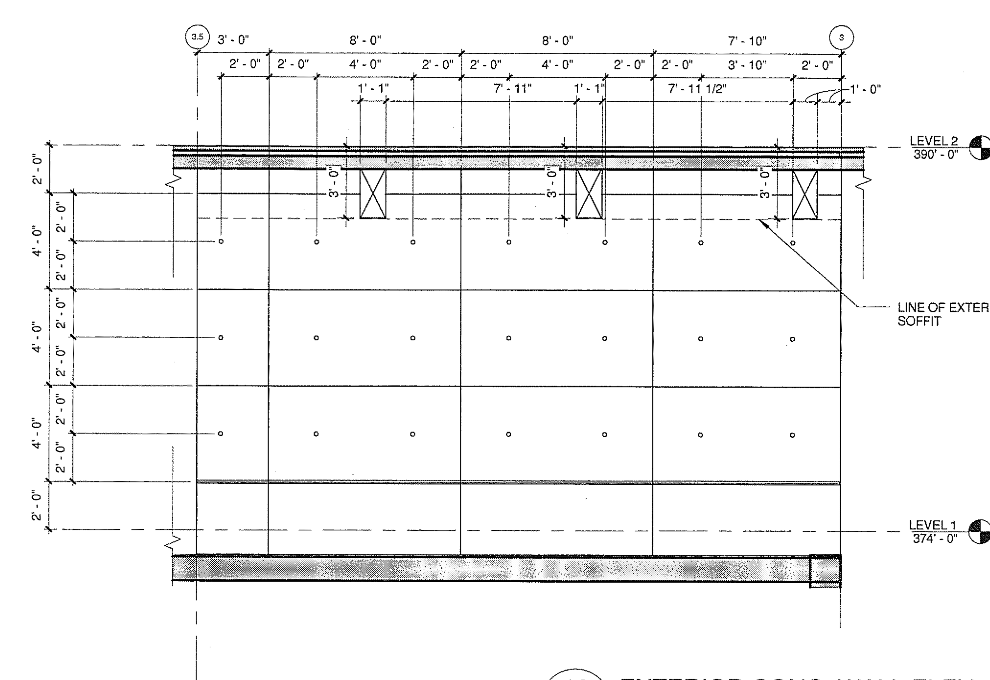
18 EXTERIOR CONC. WALL ELEV A2513 | A5320 1/4" = 1'-0"
