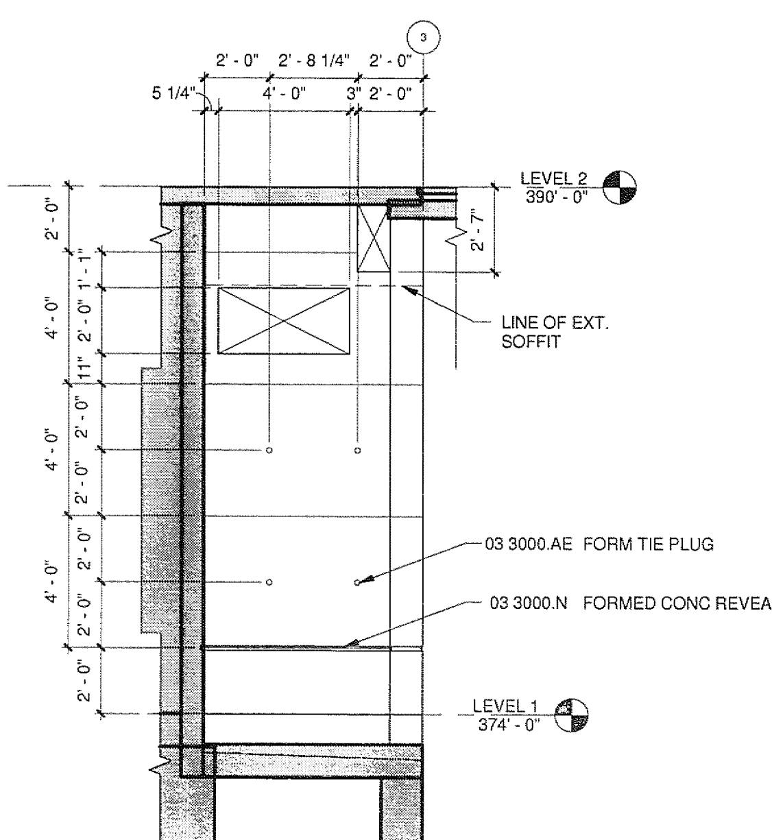
13 EXTERIOR CONC. WALL ELEV. A2513 A5320 1/4" = 1'-0"
