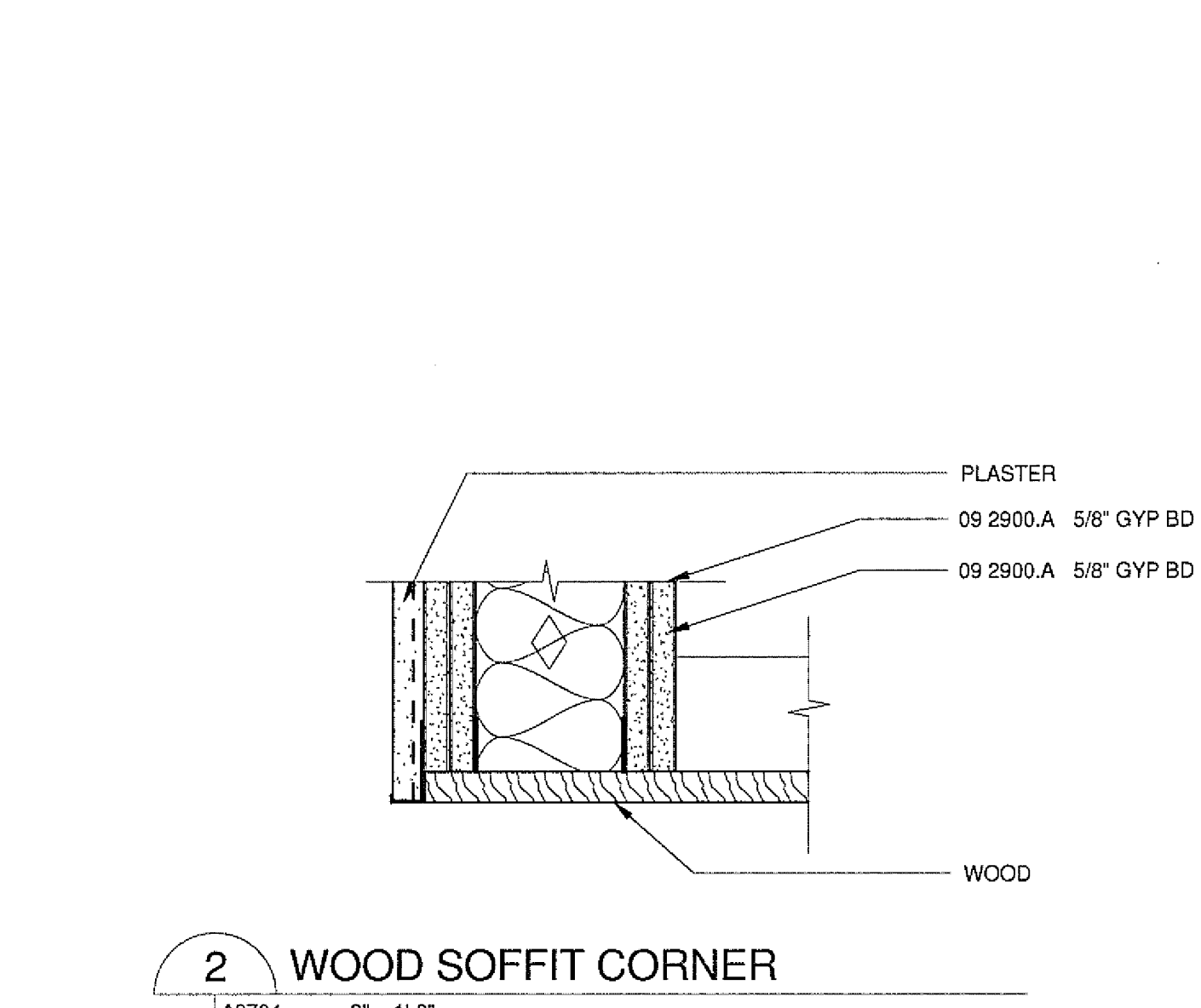
2 WOOD SOFFIT CORNER A9704 3\"/>
