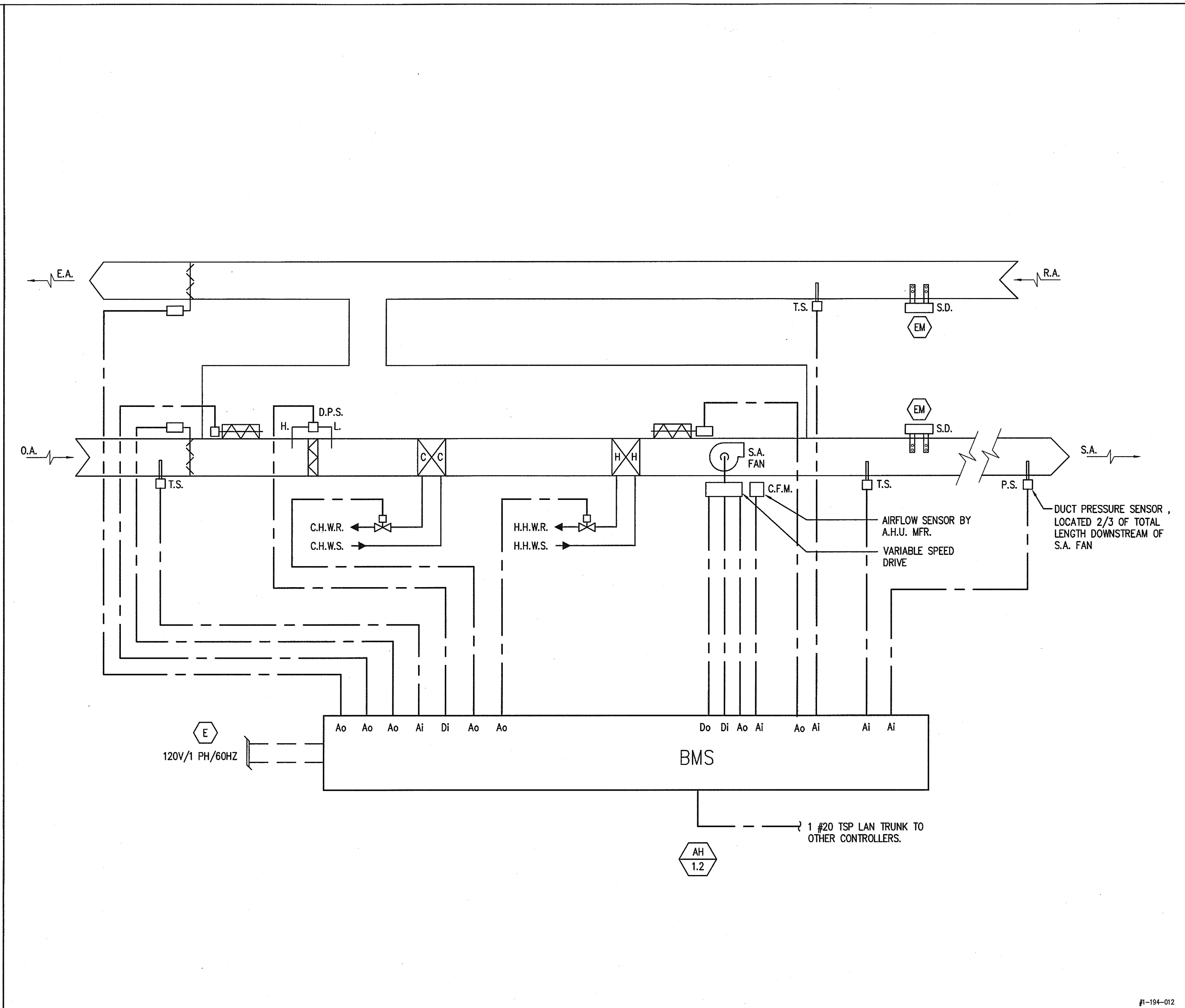
AUDITORIUM VAV A.H. UNIT (W/ FAN V.F.D.) CONTROL
