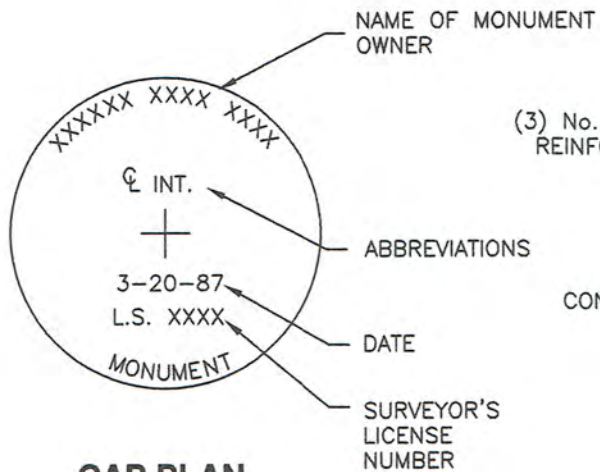
CAP PLAN
