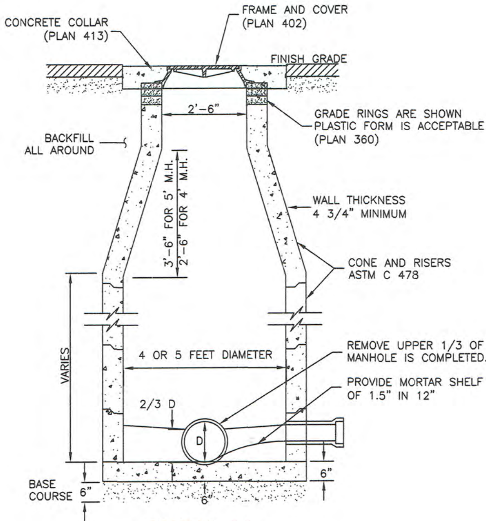
SECTION A-A
