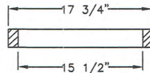
SECTION D-D
