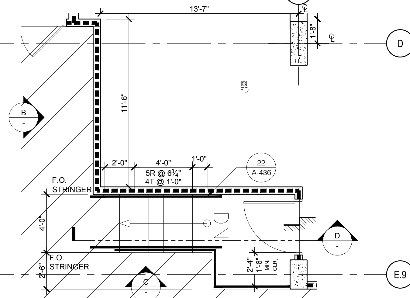
EXTERIOR STAIR (ES-3)
