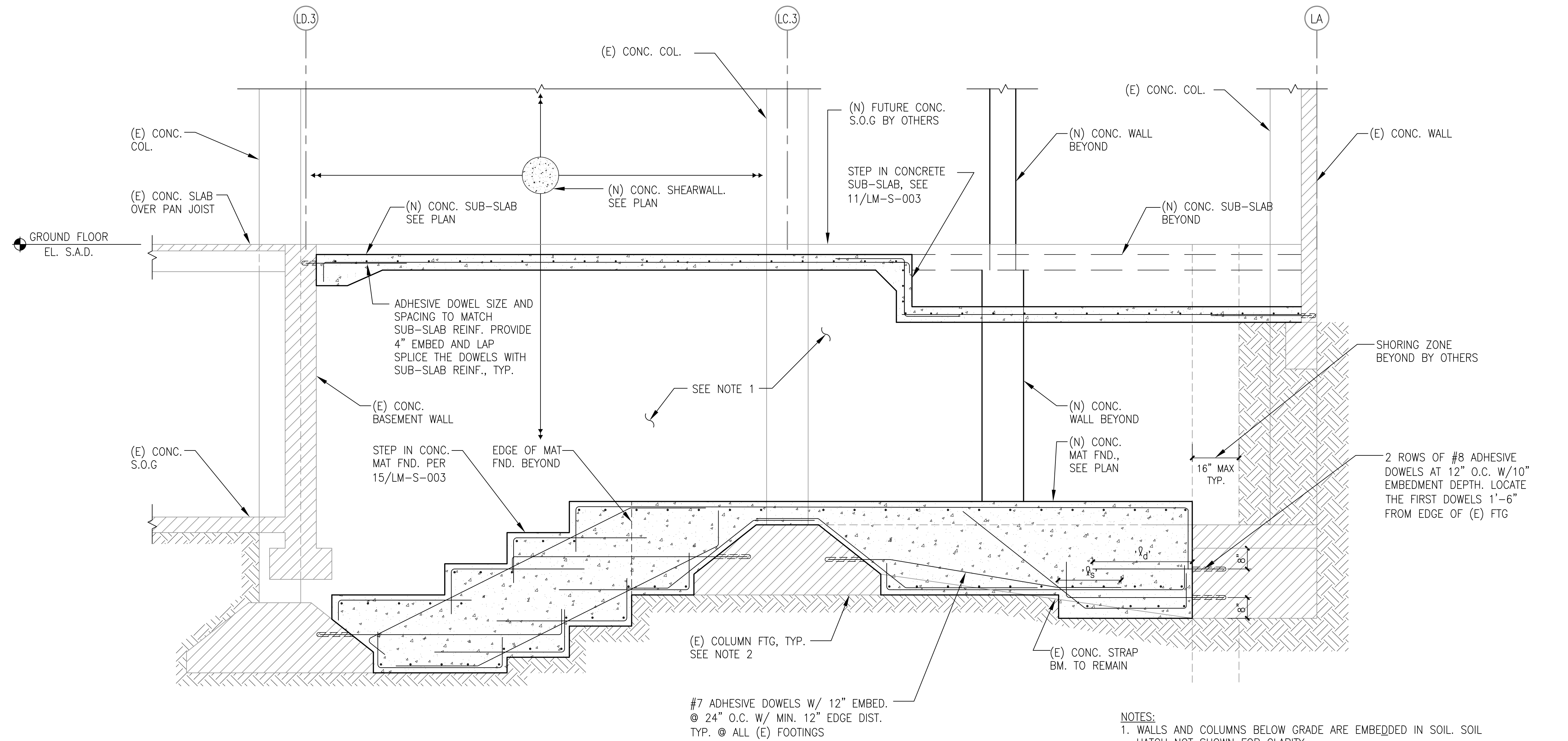
12 SECTION THRU MAT FOUNDATION N.T.S.
